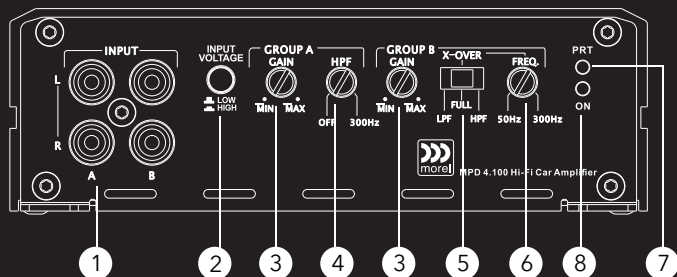
MPD 4.100 - Front panel
